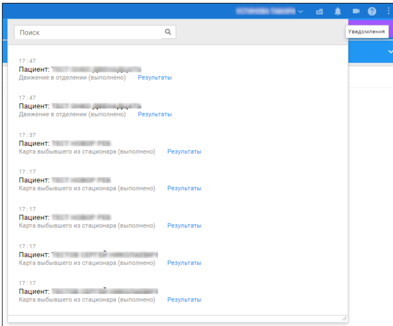
Рисунок 8 – Форма "Уведомления"
